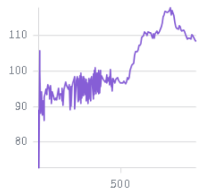
time/exclusive...pute_gradients
