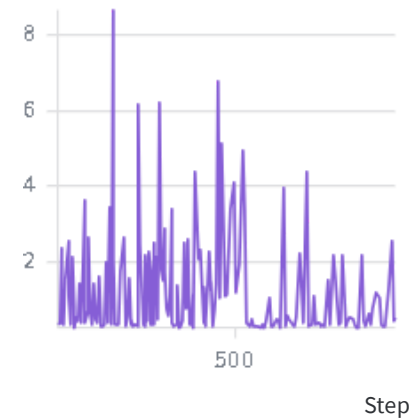
memory/mb_p...odel_backward
