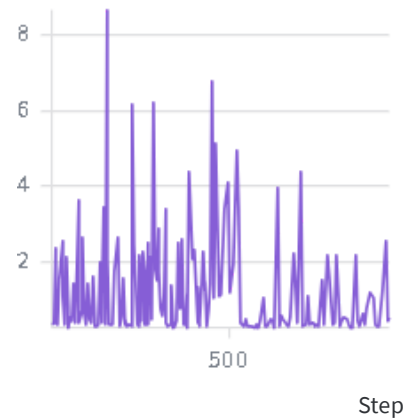
memory/mb_p...optimizer_step
